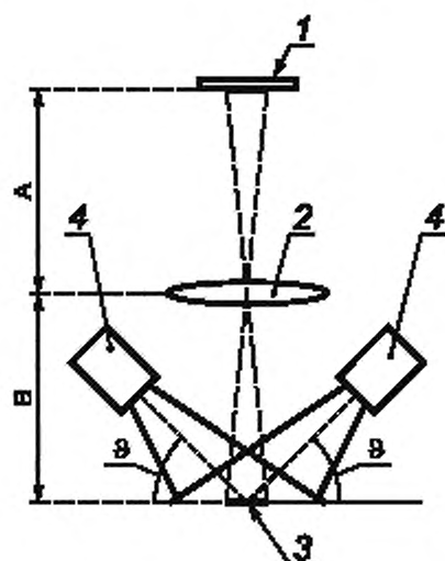
1 — светочувствительный элемент, 2 — объектив с увеличением 1.1 (расстояние A равно расстоянию B); 3 — область проверки; 4 — источник излучения; \varphi — угол падения пучка светового излучения к плоскости символа (по умолчанию — 45^\circ , допускается — 30^\circ , при диффузном излучении — 90^\circ )
