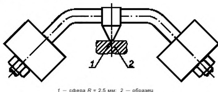
Рисунок 1 — Устройство для проверки вдавливанием шарика
