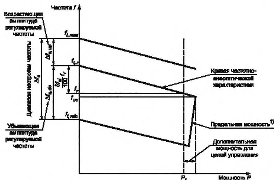
Рисунок 1 — Частотно-энергетическая характеристика диапазона регулируемой частоты
