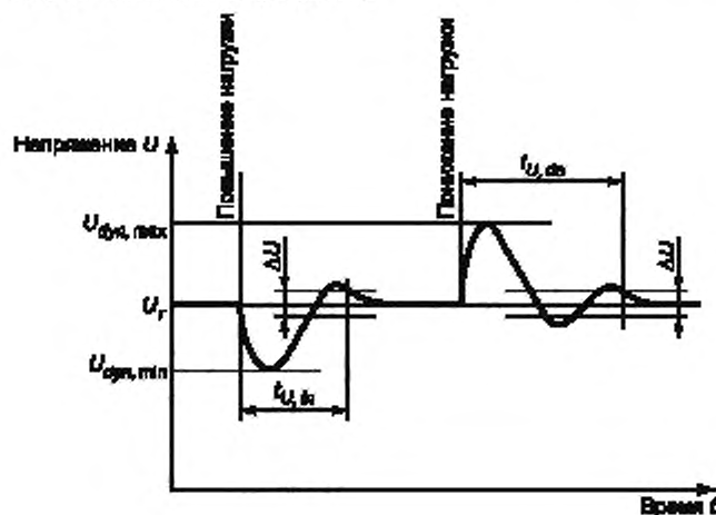
Рисунок 5 — Характеристики кратковременного напряжения без квадратурного статического отклонения напряжения компенсации
