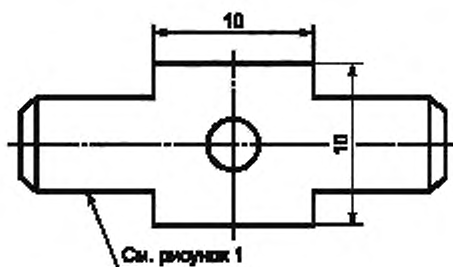
Рисунок 6 — Двухконцевой штекер
