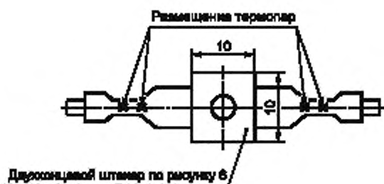
Рисунок 7 — Размещение термодпар при испытаниях
