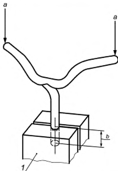
Рисунок 12 — Испытание на кручение узла руль — стержень
