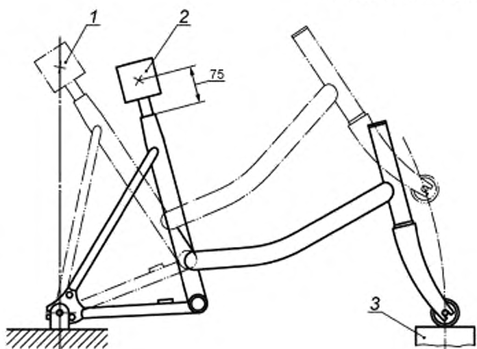
Рисунок 15 — Испытание на удар (падающий узел рамы — вилка)
