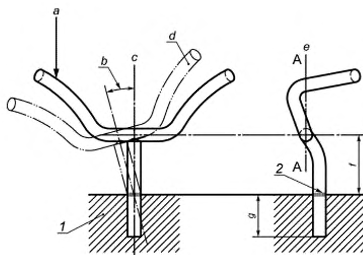
1 — зажимное приспособление; 2 — ограничительная метка, а — прикладываемый момент кручения; b — остаточная деформация, c — ось стержня; d — отклонение формы; e — прикладываемый момент кручения в сечении А—А; f — длина свободного стержня; g — минимальная глубина ввода
