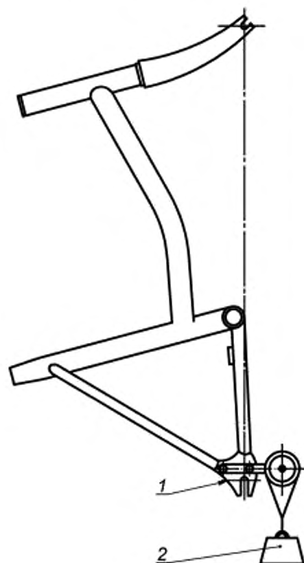
1 — рама, жестко закрепленная в вертикальном положении; 2 — масса 30 кг, действующая через ось поддерживающего ролика
