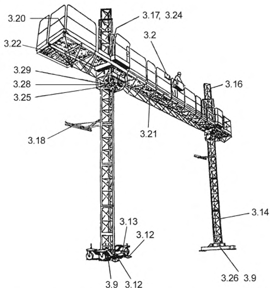
Рисунок 2 — Стандартный двухмачтовый ПРПМ
