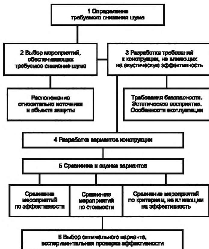
Рисунок 6 — Основные этапы проектирования шумозащитных мероприятий
