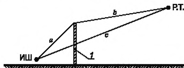
1 — экран; ИШ — источник шума; Р.Т. — расчетная точка
