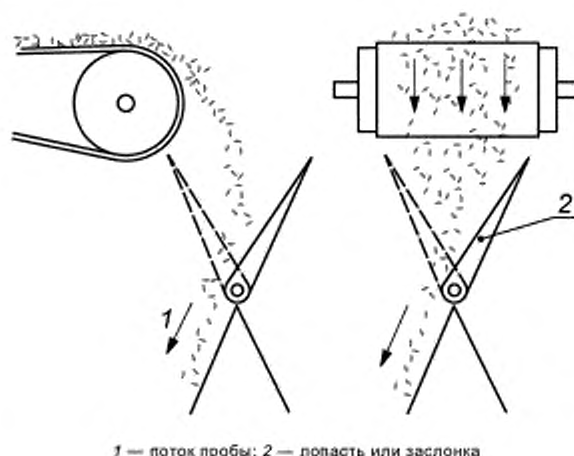
Рисунок А.4 — Пробоотборник с отклонением всего потока
