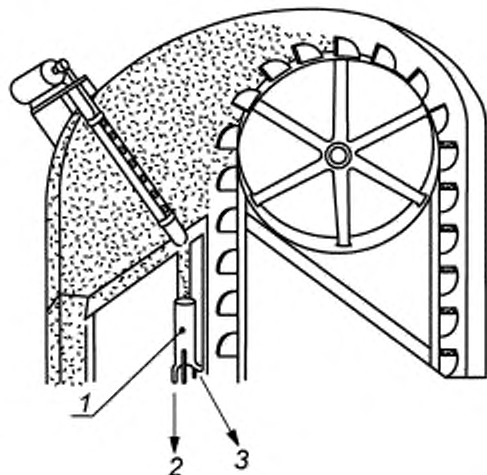
Рисунок А.1 — Поперечный пробоотборник для открытого самотека, обеспечивающий периодический и непрерывный отбор проб
