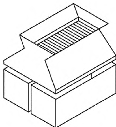
Рисунок В.14 — Многочелюбковый делитель с перегородками, пластинами и двумя ящиками для сбора пробы
