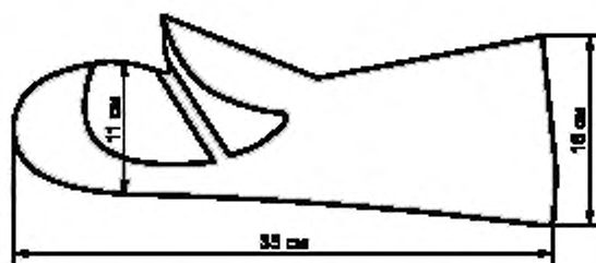
Рисунок 2 — Внутренние минимальные размеры ЗАЩИТНЫХ РУКАВИЦ
