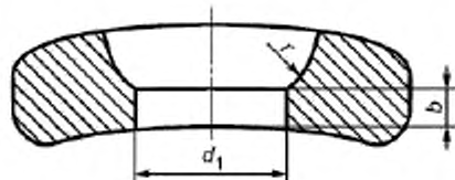
Рисунок 5 – Отверстие типа D2
