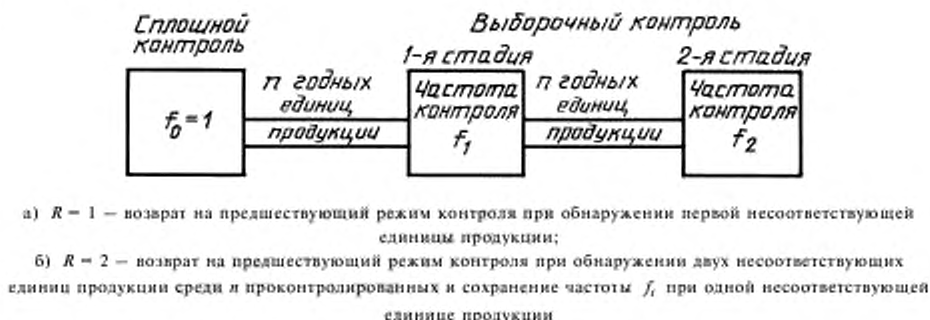
Рисунок 2 — Схема двухстадийного плана непрерывного контроля
