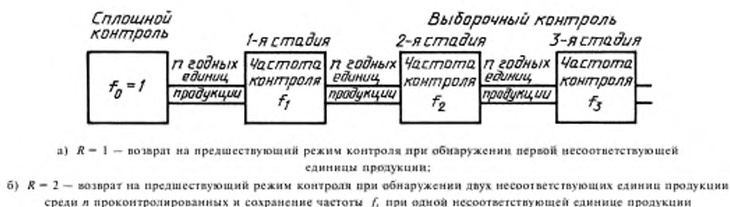
Рисунок 3 — Схема трехстадийного плана непрерывного контроля
