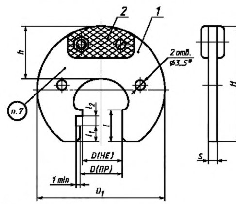
Калибры-скобы односторонние для диаметров св. 10 до 100 мм
