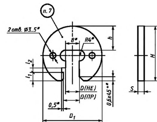
Калибры-скобы односторонние для диаметров от 3 до 10 мм
