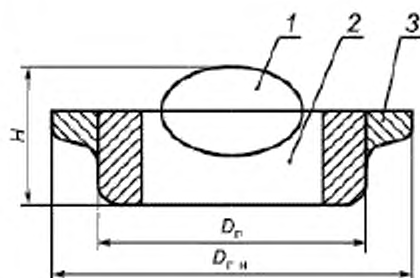
1 — запирающий элемент; 2 — проходное отверстие; 3 — фланец пришивного кольца, H — высота ПКС, D_п — посадочный диаметр ПКС; D_{г.н} — пришивной наружный диаметр ПКС
