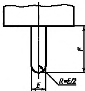
Рисунок 18 — Испытательный цокль для испытания патронов Fa6 по разделу 13
