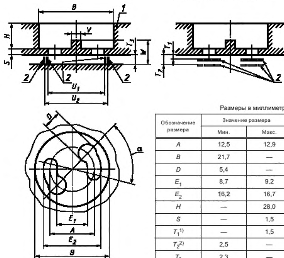
Вариант расположения контактов
