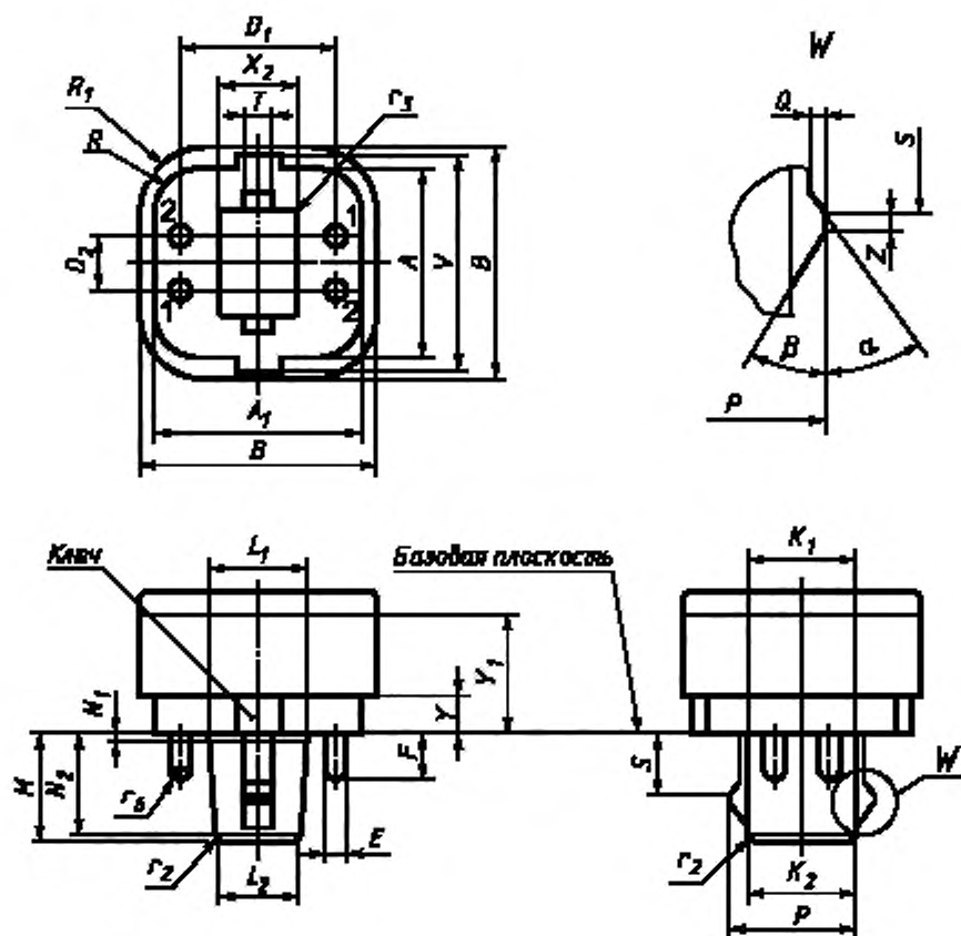
Рисунок 37 — Испытательный цоколь для испытания патронов G24, GX24 и GY24 по 17.1
