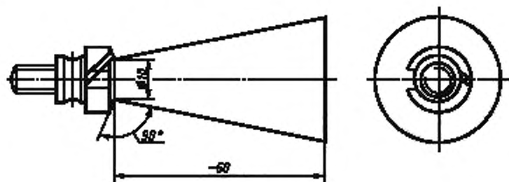
Рисунок 1 — Коническая оправка
