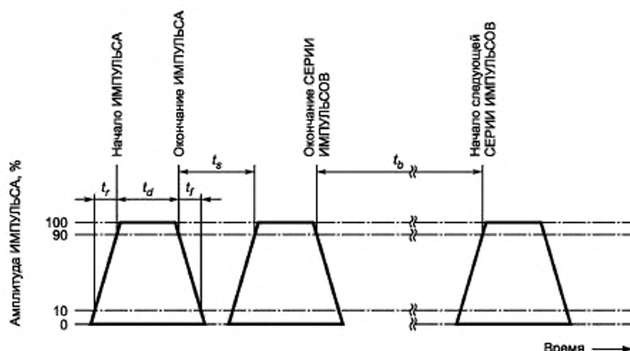
Рисунок 201 – Пояснение временных характеристик звуковых СИГНАЛОВ ОПАСНОСТИ
