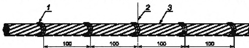
1 — проволоочный бандаж; 2 — центр; 3 — число отрезков, равное семи
