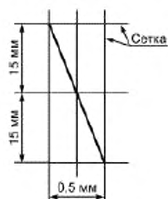
Рисунок 109 – Проверка прямоугольности системы координат (см. 51.108.4.1)
