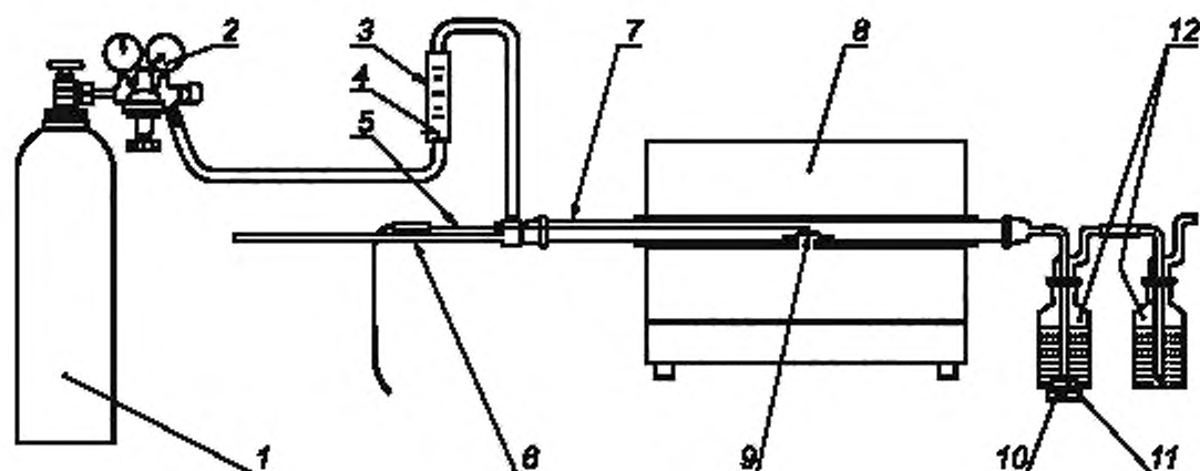
1 — баллон с искусственным воздухом; 2 — редуктор; 3 — ротаметр; 4 — игольчатый вентиль; 5 — термопара; 6 — устройство для ввода подложки с образцом; 7 — трубка из кварцевого стекла; 8 — печь; 9 — лодочка с образцом; 10 — магнитная мешалка; 11 — стержень магнитной мешалки; 12 — промывочные сосуды
