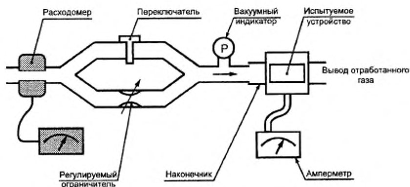
Рисунок 7 – Испытание передвижного отсасывающего устройства, работающего от батареи
