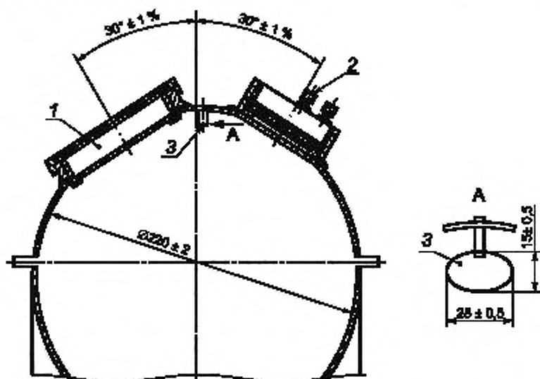
1 — апертура фары; 2 — фотозлемент; 3 — дефлектор; А — увеличение (расширение) дефлектора (вид в направлении стрелки)
