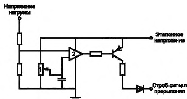
1 — устройство регулирования скорости переключения; 2 — блок сравнения
