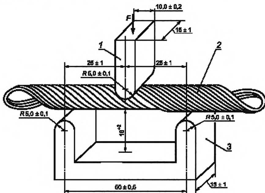
1 — ползун; 2 — макет обмотки; 3 — подставка, F — усилие
