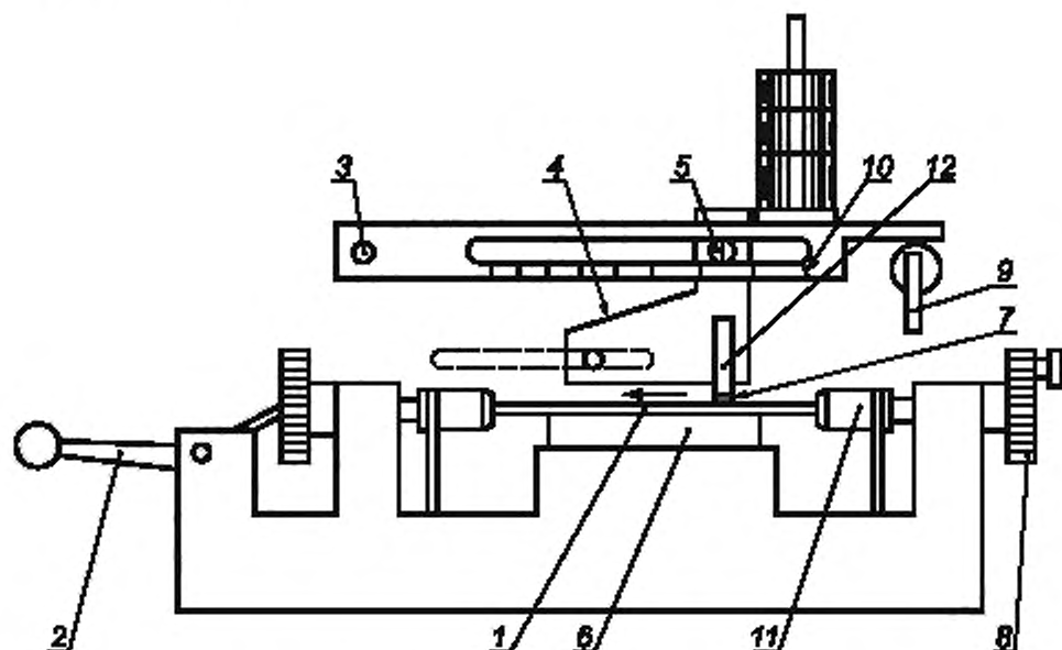
1 — образец; 2 — натяжное устройство для распрямления образца; 3 — фиксированная точка вращения; 4 — нагруженное истирающее устройство; 5 — указатель; 6 — опора, перемещающаяся по высоте; 7 — рессорная проволока; 8 — планшайба для поворота на 120^\circ ; 9 — рычаг возврата в исходное положение; 10 — градуированная шкала, на которой отмечают коэффициент умножения; 11 — зажим; 12 — скребок
