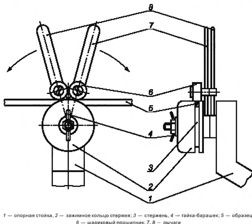
Рисунок 4 — Устройство для испытания намоткой на стержень
