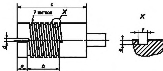
Рисунок 2 — Конструкция и размеры оправки
