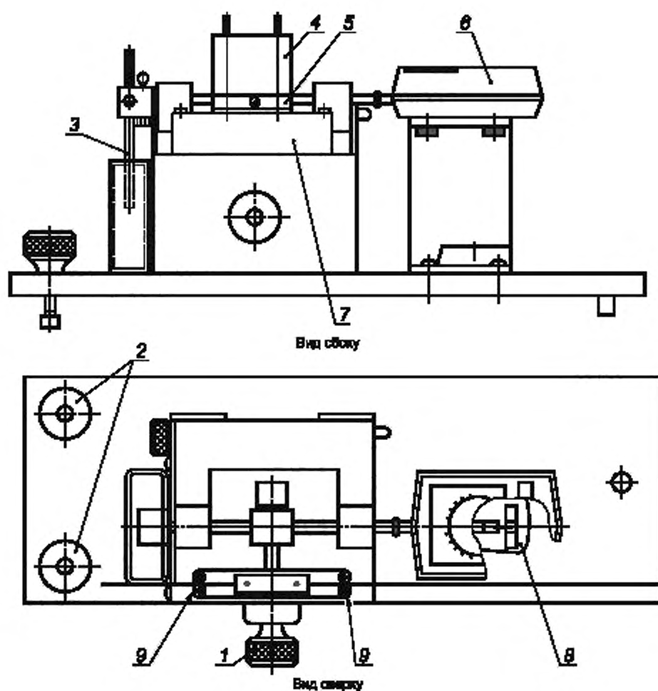
1 — регулировочное устройство; 2 — регулировочные винты; 3 — система амортизации; 4 — испытательный груз; 5 — блок нагрузки (см. рисунок В.5); 6 — динамометр; 7 — плита; 8 — поплавковый уровень; 9 — направляющие
