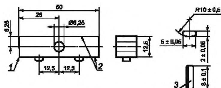
1 — притупленные углы; 2 — поверхности плоские и параллельные; 3 — искусственный сапфир
