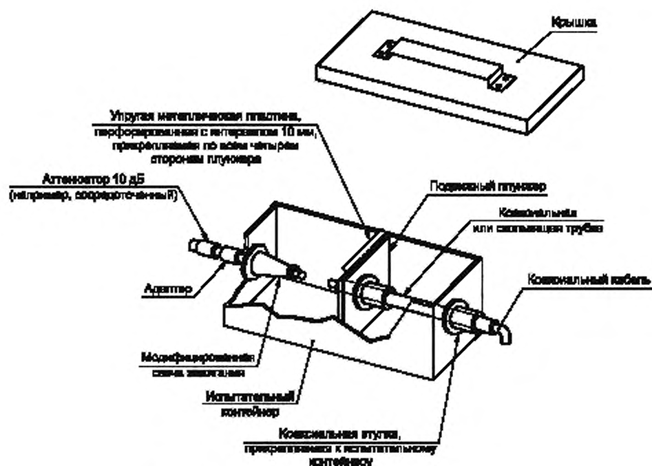
Рисунок Е.2 — Общий вид испытательного контейнера
