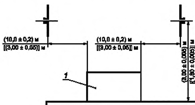
Рисунок 7 — Расположение антенны при измерении излучаемых радиопомех — вертикальная поляризация
