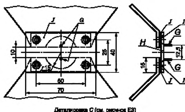
Детализация C (см. рисунок E3)
