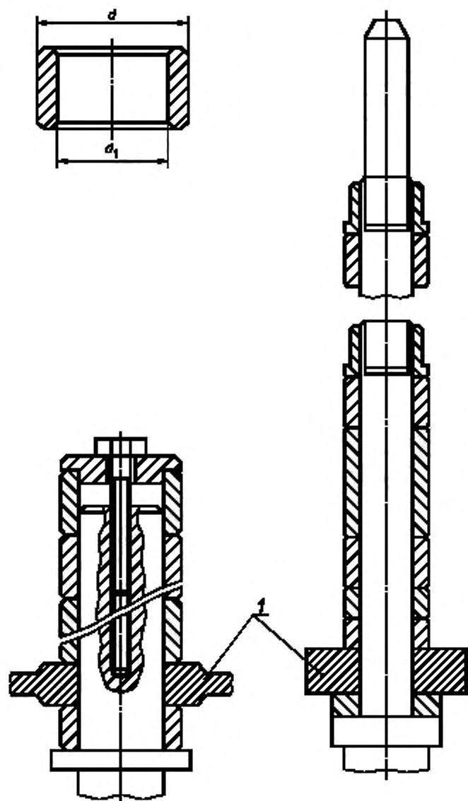
Рисунок 102 — Шпindel резцедержателя и дистанционные кольца шпинделя
