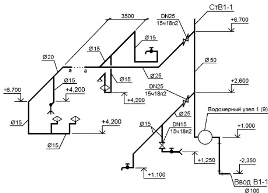
Рисунок Б.1 — Пример выполнения схемы системы водоснабжения
