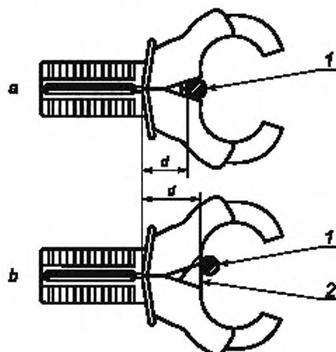
а — без устройства защиты проводника; б — с устройством защиты проводника, 1 — проводник; 2 — устройство защиты проводника
