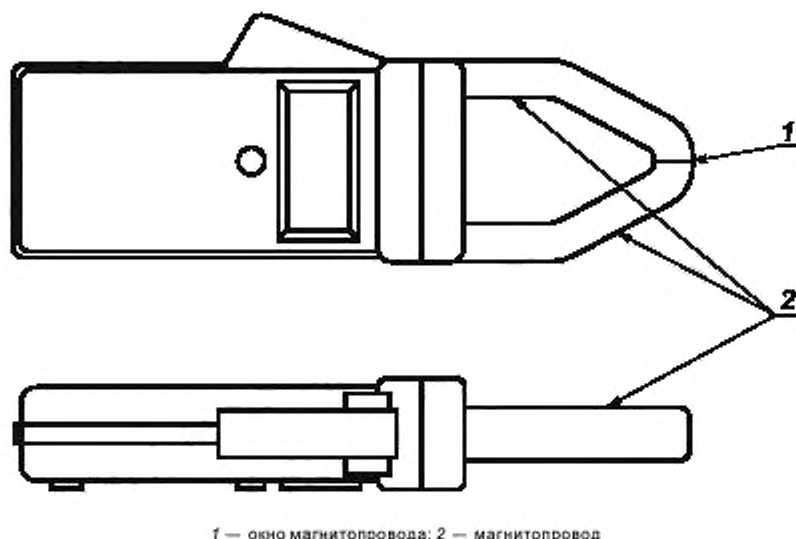
Рисунок 102 — Пример амперометрических клещей, применяемых в качестве оборудования согласно IEC 61010-1
