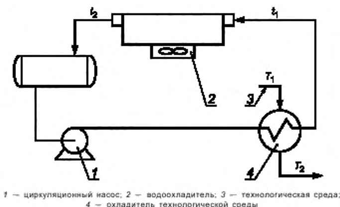
Рисунок С.12 — Система с промежуточной водой
