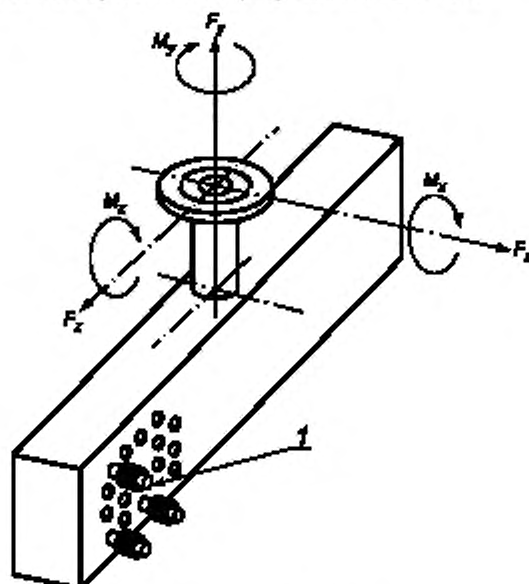
Рисунок 6 — Нагрузки на патрубки
