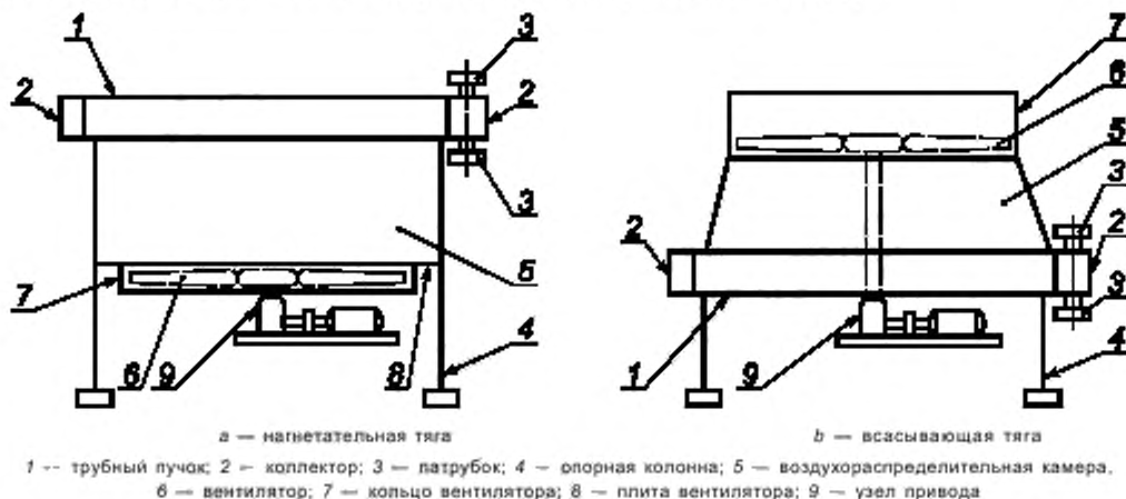
Рисунок 2 — Типичные элементы аппарата с воздушным охлаждением
