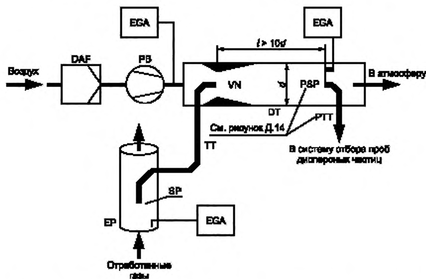
Рисунок Д.8 — Система с частичным разбавлением потока, частичным отбором проб, одинарной трубкой Вентури и измерением концентрации \text{CO}_2 и \text{NO}_x
