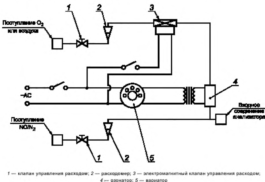
Рисунок Д.1 — Схема устройства для проверки эффективности преобразователя \text{NO}_2 в \text{NO}
