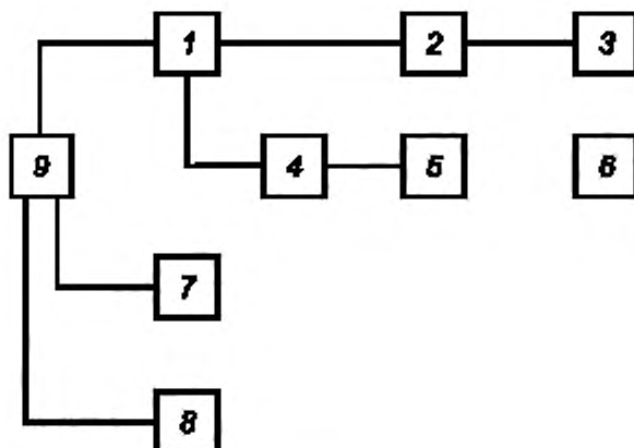
1 — аллифазометр; 2, 4 — фазостабилизированные СВЧ кабели; 3 — антенна НАП; 5 — излучающая антенна; 6 — эталонная антенна; 7 — устройство управления ОПУ; 8 — устройство управления УЛП; 9 — персональный компьютер
