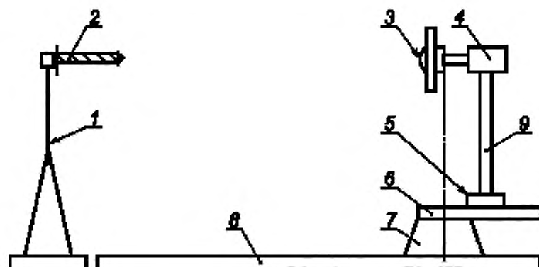
1 — опора; 2 — излучающая антенна; 3 — антенна НАП; 4 — ОПУ по углу \varphi ; 5 — лоперечная каретка; 6 — продольная каретка; 7 — ОПУ по углу \theta ; 8 — УЛП; 9 — мачта
