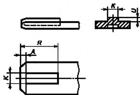
Рисунок Е.12 — Размеры штыревого наконечника
