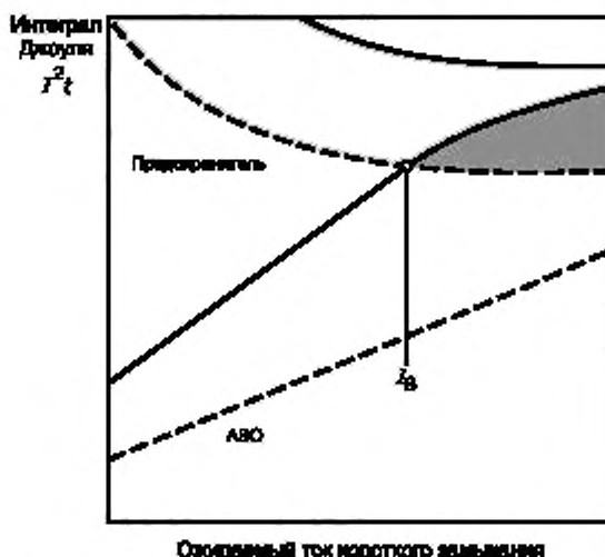
Рисунок F.6 — Токоограничивающий АВР, защищаемый автоматическим выключателем с тепловой и электромагнитной защитой
