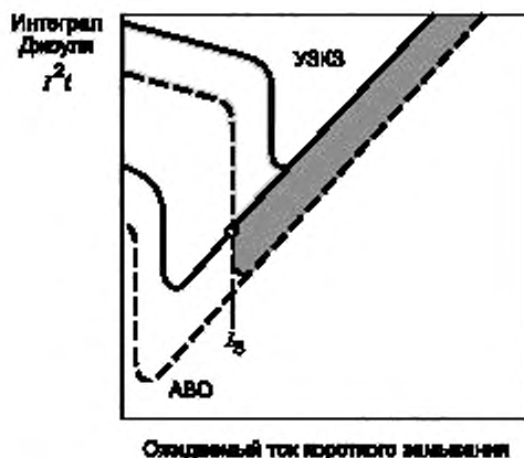
Ожидаемый ток короткого замыкания
