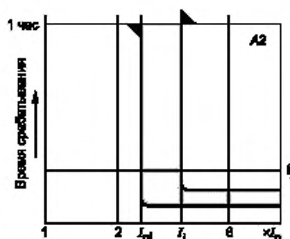
Рисунок А.2 — Характеристика только электромагнитной защиты
