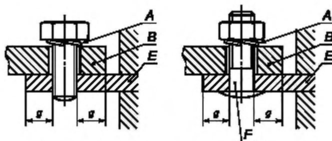
А — устройство против самоотвинчивания; В — кабельный наконечник или шина; Е — неподвижная часть; F — винт; g — расстояние перекрытия
