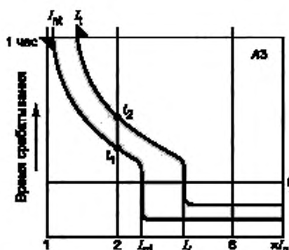
Рисунок А.3 — Характеристика тепловой и электромагнитной защиты
