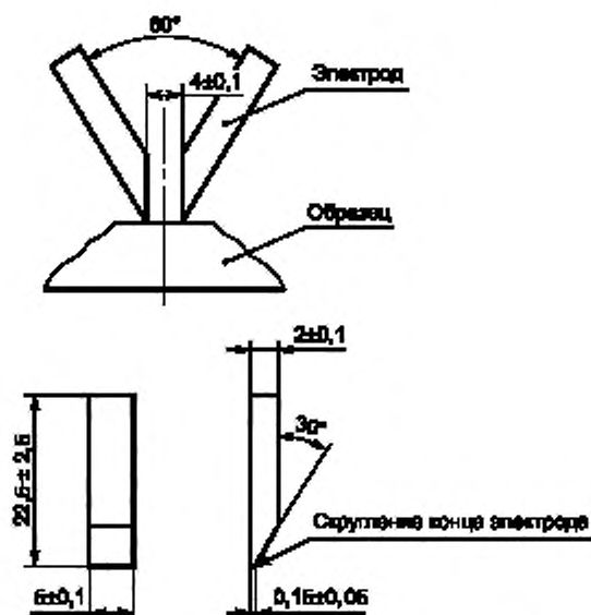
Рисунок 9 — Расположение и размеры электродов для испытания на трещиностойкость
