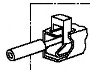
Рисунок E.5 — Примеры безрезьбовых выводов
