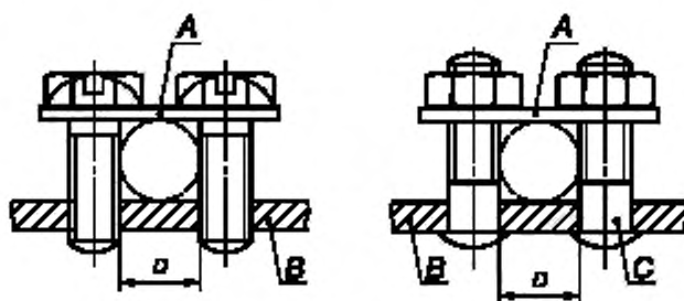
A — планка; B — неподвижная часть; C — винт; D — окно для проводника
