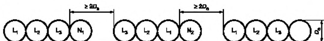
Рисунок Н.52.4 — Специальная конфигурация для девяти параллельных одножильных кабелей в горизонтальной плоскости (см. 523.7)
