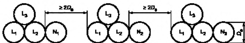
Рисунок Н.52.6 — Специальная конфигурация для девяти параллельных одножильных кабелей, уложенных треугольником (см. 523.7)
