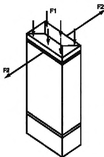
F1 — равномерно распределенная нагрузка 8500 \text{ Н/м}^2 ; F2 — растягивающие усилия 1200 Н
