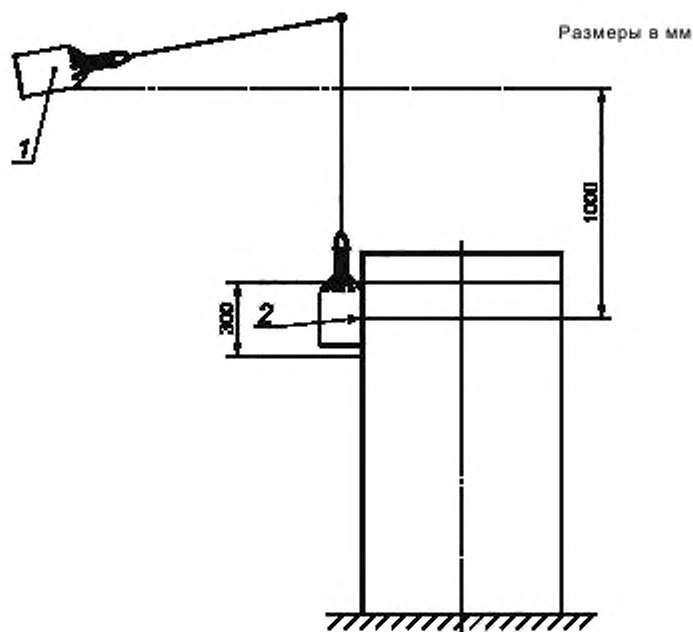
б — Схема испытания по проверке устойчивости ЩРКП — И к ударной нагрузке
