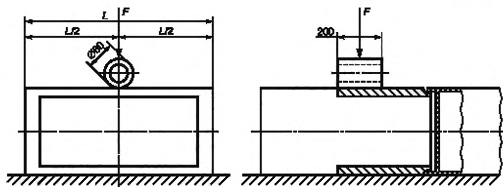
Рисунок 110 — Схема испытания для проверки механической прочности основания
