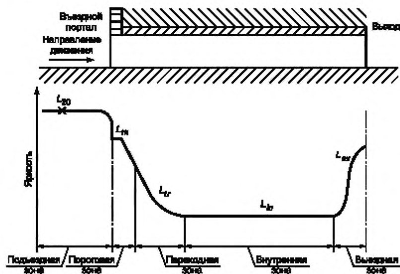
Рисунок Б.4 — Схема расположения яркостных зон в туннеле ( L_{20} , L_{2r} , L_{2l} , L_{2tr} , L_{2tl} , L_{2ex} — по [1])
