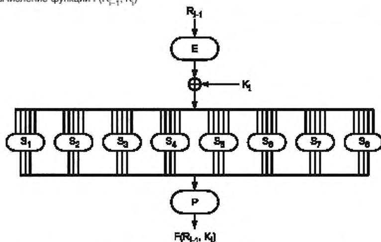
В.2.1.2 Вычисление функции f(R_{i-1}, K_i)
