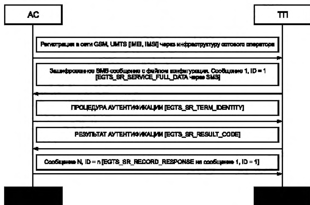
Рисунок 4 — Алгоритм конфигурации АС с использованием SM
