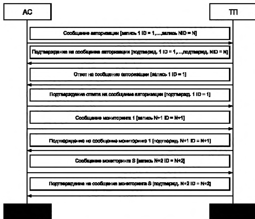
Рисунок 3 — Диаграмма обмена сообщениями
