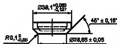
Рисунок 5 — Втулка держателя пробы
