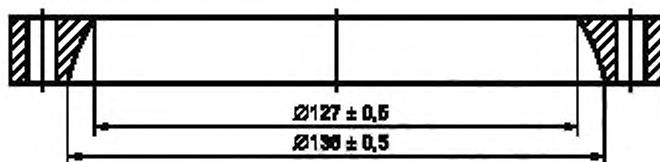
Рисунок 2 — Прижимное кольцо
