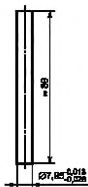
Рисунок 3 — Ось держателя пробы
