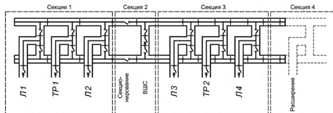
Рисунок Б.3 — Однолинейная электрическая схема и схема подразделения на газовые отсеки
