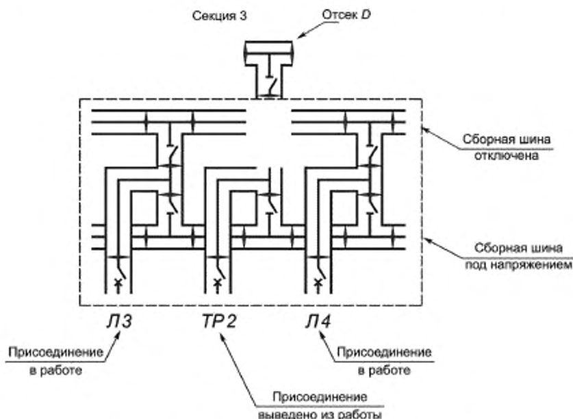
Рисунок Б.6 — Демонтаж шинного разъединителя в секции 3
