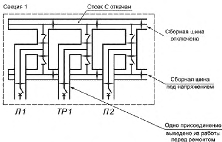
Рисунок Б.4 — Локализация и изоляция
