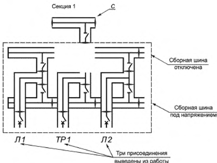
Рисунок Б.5 — Демонтаж шинного разъединителя в секции 1
