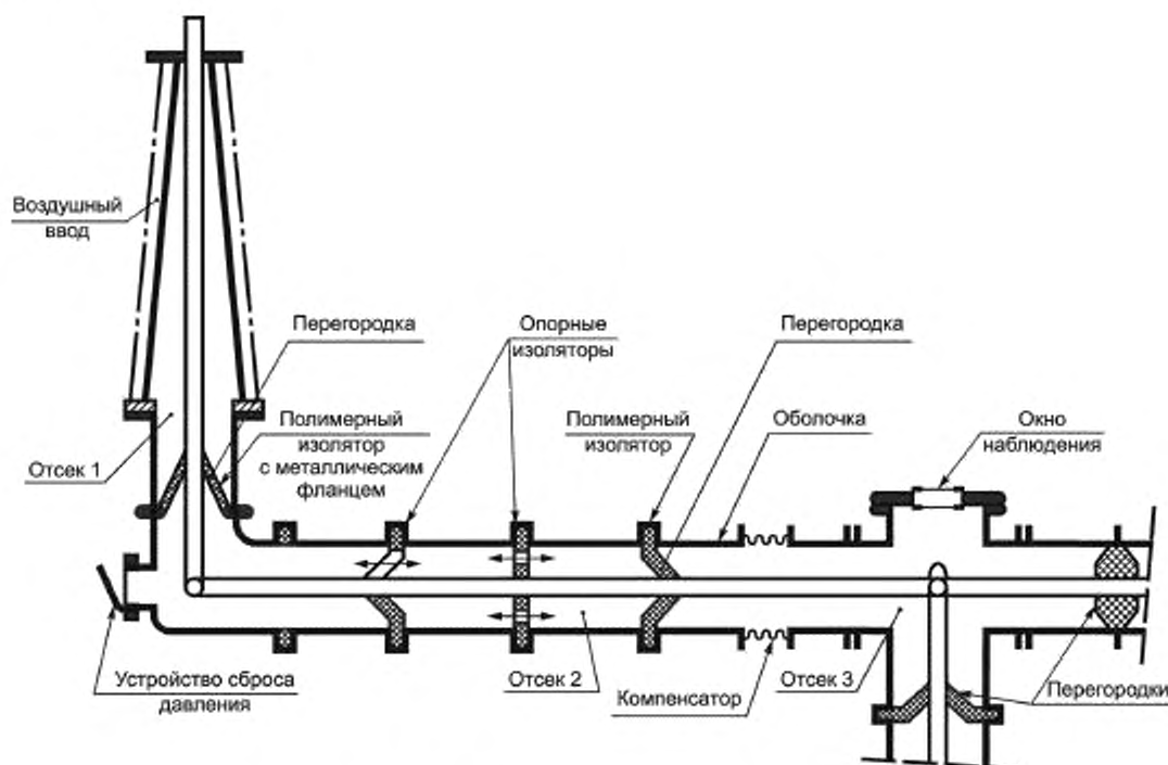
Рисунок 3 — Пример расположения оболочек и газовых отсеков
