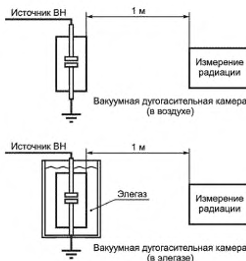
Рисунок 5 — Место монтажа дозиметра
