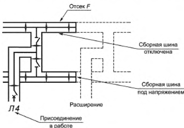
Рисунок Б.7 — Расширение КРУЭ
