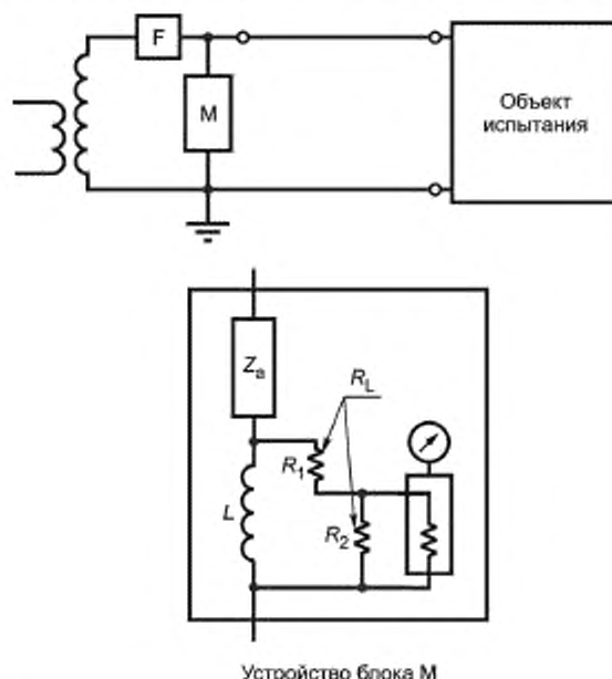
Устройство блока М
