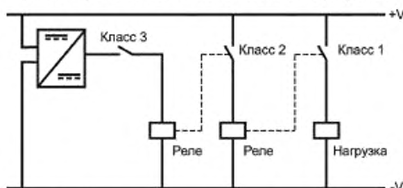
Рисунок 1 — Примеры классов контактов
