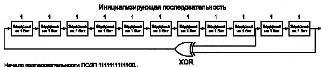
Рисунок 8 — Схема генератора опорной последовательности
