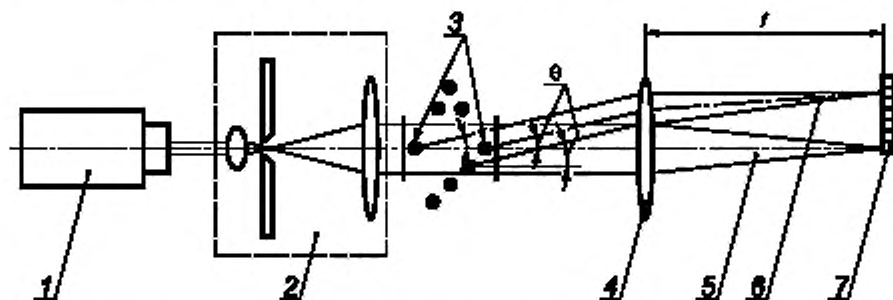
1 — источник электромагнитного излучения (лазер); 2 — блок формирования луча (расширитель); 3 — частицы, взвешенные в образце; 4 — линза; 5 — нерассеянный пучок; 6 — рассеянное излучение; 7 — многоэлементное фотоприемное устройство; θ — угол рассеяния; f — фокусное расстояние линзы
