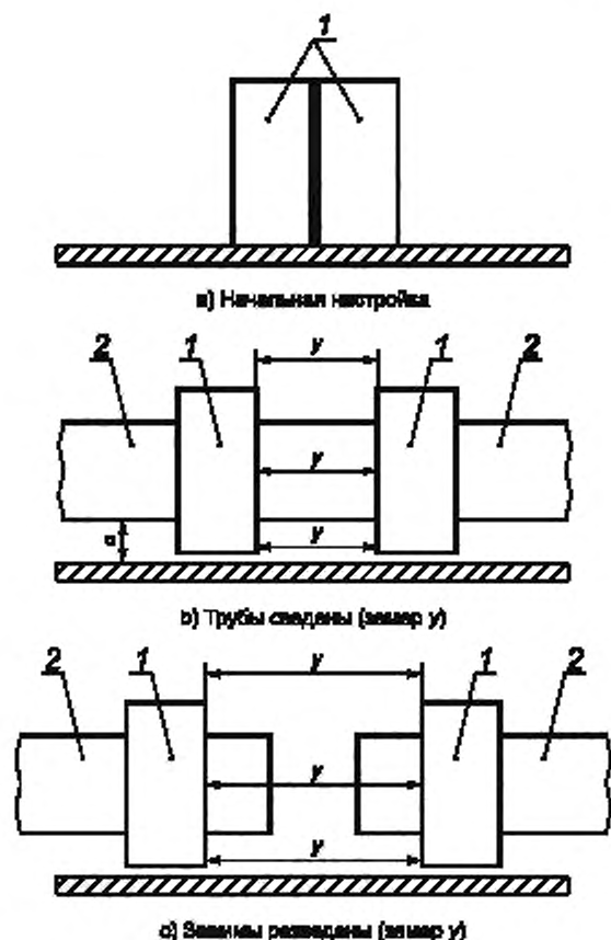
Рисунок 4 — Испытания на подтверждение центрирующей способности зажимов
