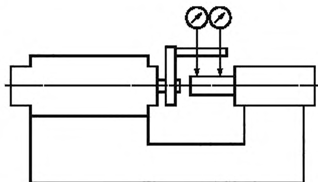
Рисунок А.1 — Измерение соосности внешней осевой нагрузки
