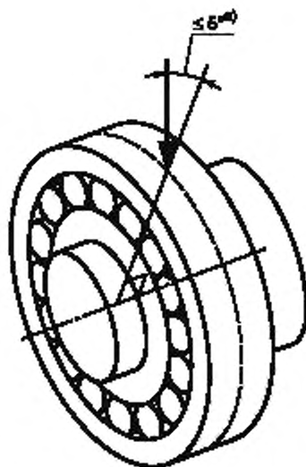
Рисунок 3 — Отклонение от радиальной оси (ИСО 15242-3:2006/Попр.1:2010)
