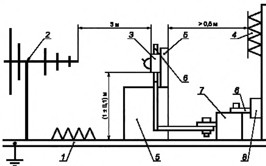
1 — заземляющая пластина; 2 — антенна; 3 — испытываемый аппарат; 4 — поглотители эха; 5 — изолирующий материал; 6 — соединения, удерживаемые на минимуме; 7 — трансформатор; 8 — главный фильтр
