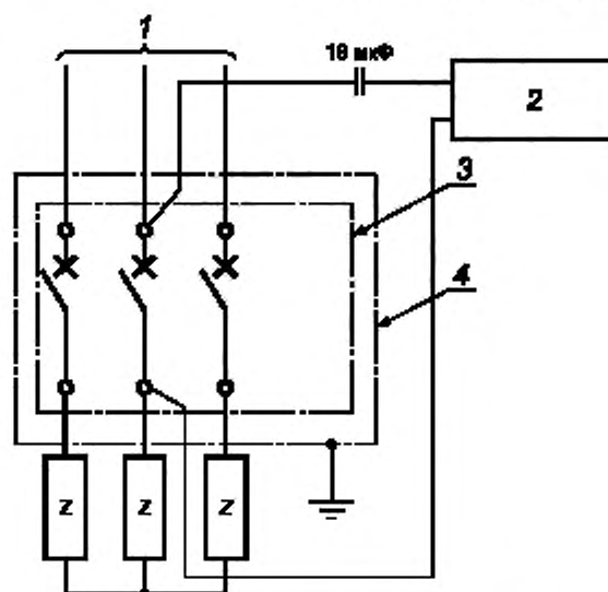
Рисунок 21 — Испытательная цепь для проверки устойчивости к влиянию импульсов в главной цепи (между фазой и землей). Трехфазная конфигурация цепи
