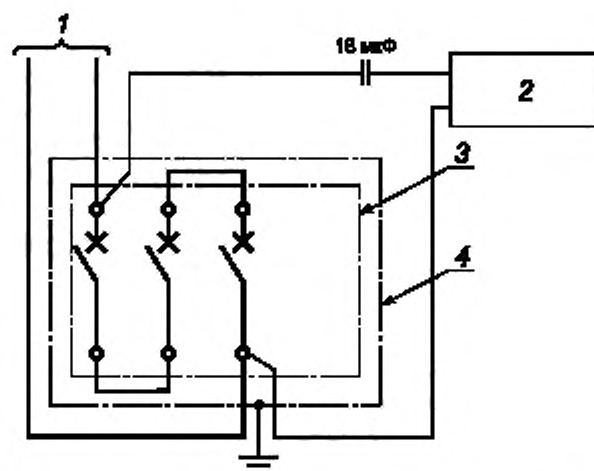
1 — источник питания; 2 — генератор импульсов; 3 — испытываемый аппарат; 4 — оболочка (по применению)
