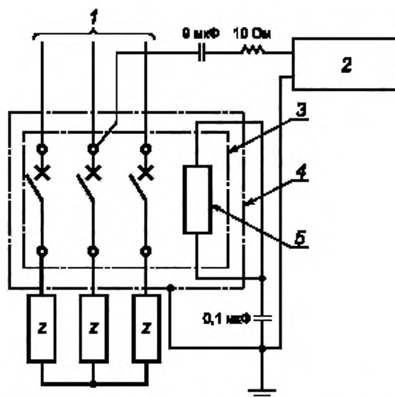
Рисунок 21 — Испытательная цепь для проверки устойчивости к влиянию импульсов в главной цепи (между фазой и землей). Трехфазная конфигурация цепи
