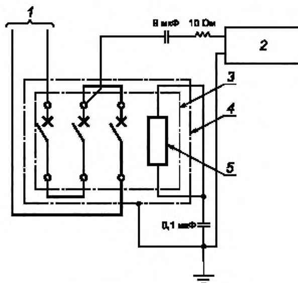
1 — источник питания; 2 — генератор импульсов; 3 — испытываемый аппарат; 4 — оболочка (по применению); 5 — вспомогательное устройство
