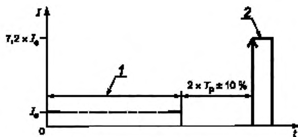
Рисунок 26 — Испытание на тепловую память
