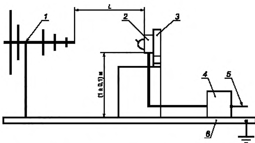
Рисунок 25 — Установка для испытания на помехозащищенность
