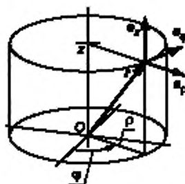
Рисунок 2 — Цилиндрическая система координат (правосторонняя)
