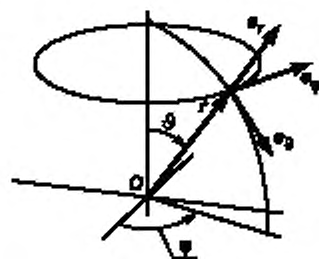
Рисунок 3 — Сферическая система координат (правосторонняя)
