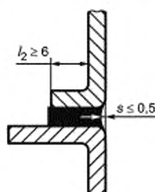
Рисунок А.14 — Зона разбрызгивания. Сварное соединение встык
