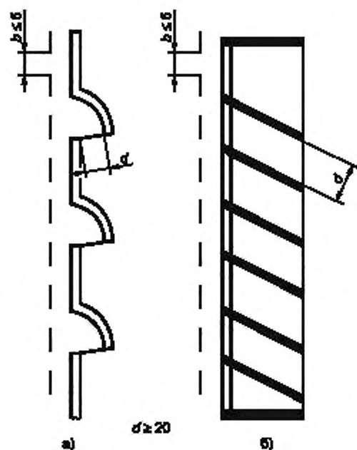
Рисунок А.19 — Вентиляционные отверстия для непищевой зоны
