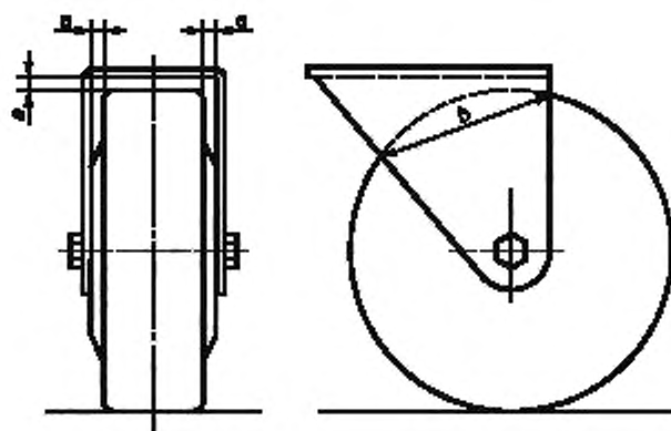
Рисунок А.18 — Пример колеса, доступного для очистки
