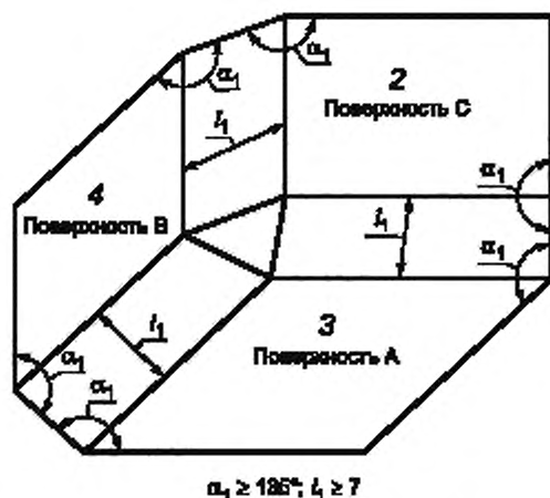
Рисунок А.4 — Пищевая зона. Три соединенные поверхности
