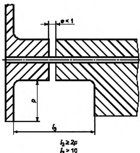
Рисунок А.20 — Шарнирное соединение
