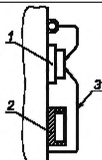
Рисунок 5 — Выключатель с защитным кожухом
