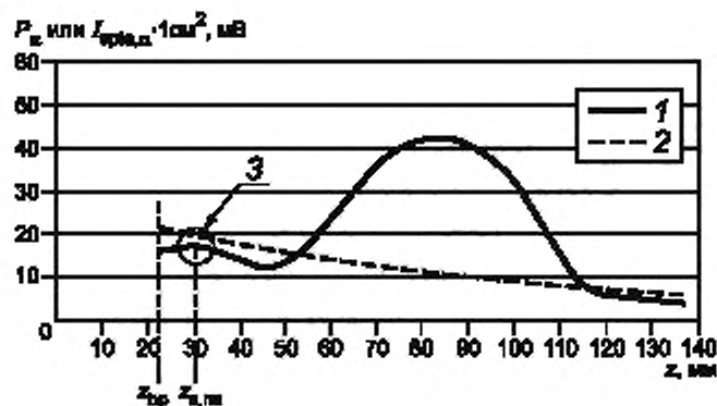
1 — график I_{ср,ср,α} \cdot 1 \text{ см}^2 ; 2 — график P_P ; 3 — точка, соответствующая P_P = I_{ср,ср,α} \cdot 1 \text{ см}^2
