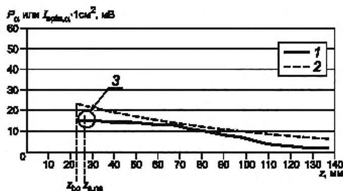
1 — график I_{ср,ср,α} \cdot 1 \text{ см}^2 ; 2 — график P_P ; 3 — точка, соответствующая P_P = I_{ср,ср,α} \cdot 1 \text{ см}^2
