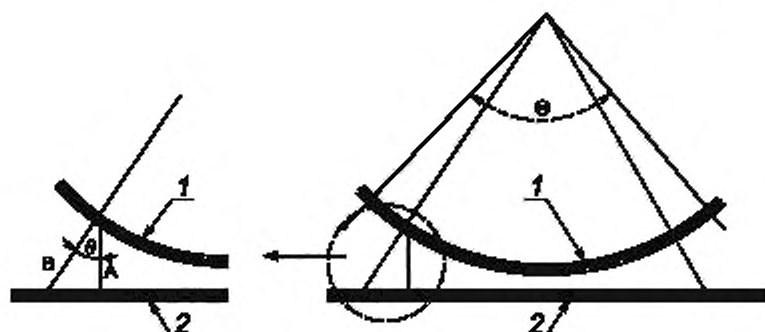
1 — решетка; 2 — поглощающая мишень; \Theta — угол сканирования; \theta — угол падения
