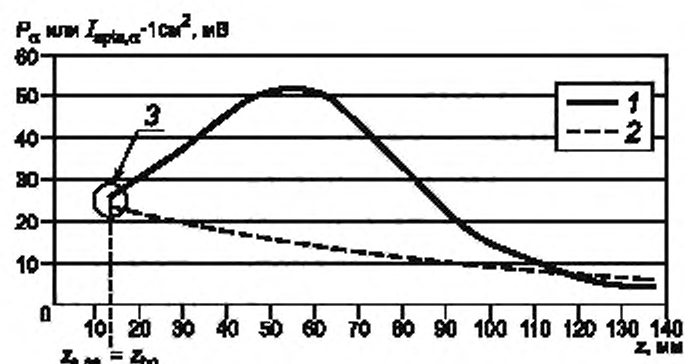
1 — график I_{spta, \alpha} \cdot 1 \text{ см}^2 ; 2 — график P_\alpha ; 3 — точка, соответствующая P_P = P_\alpha(z_{s, ns})
