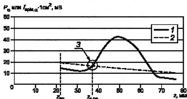
1 — график I_{spta, \alpha \times 1 \text{ см}^2} ; 2 — график P_0 ; 3 — точка, где P_0 = P_0(z_s, ns) = I_{spta, \alpha \times 1 \text{ см}^2}
