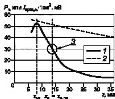
1 — график I_{spta, \alpha \times 1 \text{ см}^2} ; 2 — график P_0 ; 3 — точка с P_0 = P_0(z_s, ns) z_{Ml} расположен ближе к преобразователю, чем 1,5 \cdot D_{eq}
