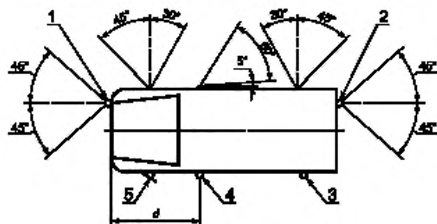
1 — передний указатель поворота; 2 — задний указатель поворота; 3 — задний боковой габаритный огонь автожелтого цвета; 4 — боковой указатель поворота; 5 — передний боковой габаритный огонь
