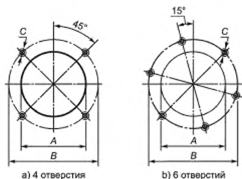
Рисунок 1 — Присоединительные размеры горелок
