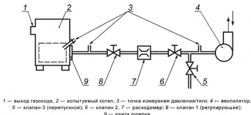
Рисунок 2 — Стенд для испытания котлов на газоплотность
