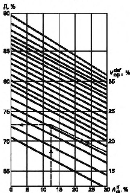
Рисунок 4 — Номограмма для определения добавки инертной пыли (D)
